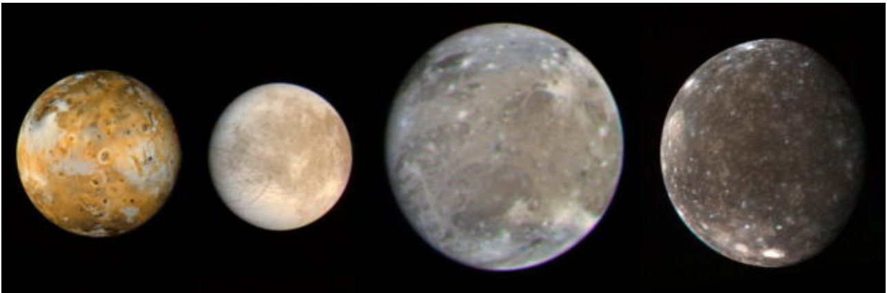
Io, Europa, Ganymed und Kallisto. NASA/JPL-Caltech, Planetary Photojournal, PIA00012
